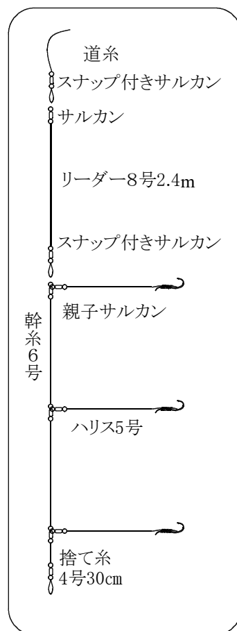
【ウタセ真鯛釣り仕掛け】
